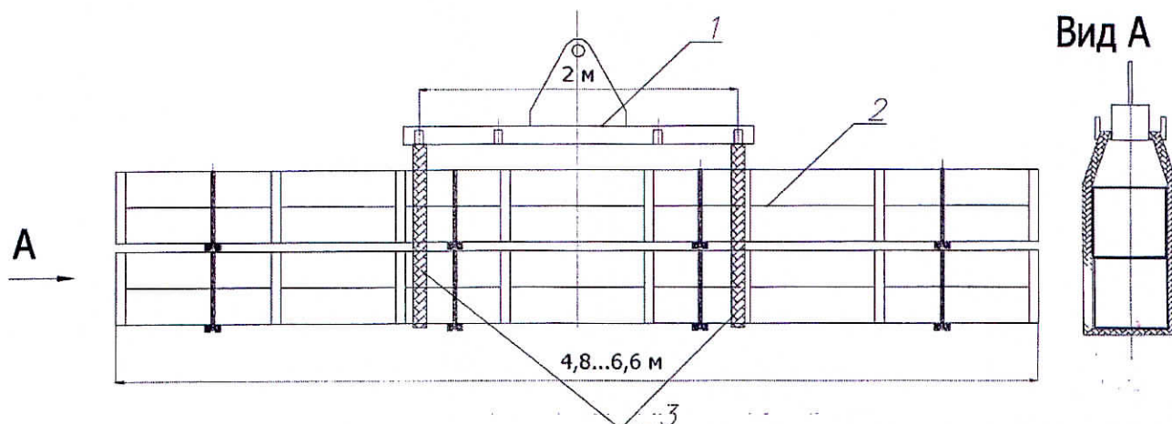
Схема строповки универсальной (балочной) траверсой
